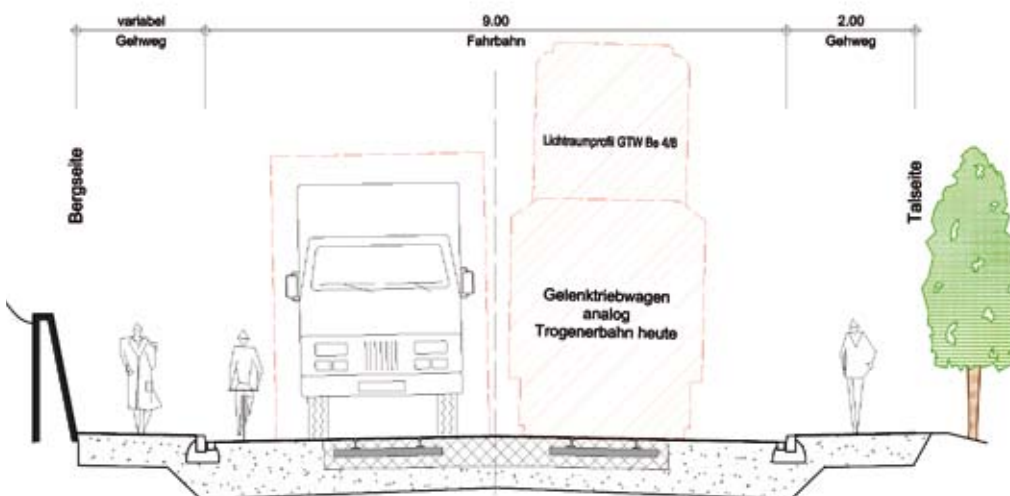
Normalprofil der geplanten Tram-Doppelspur.
