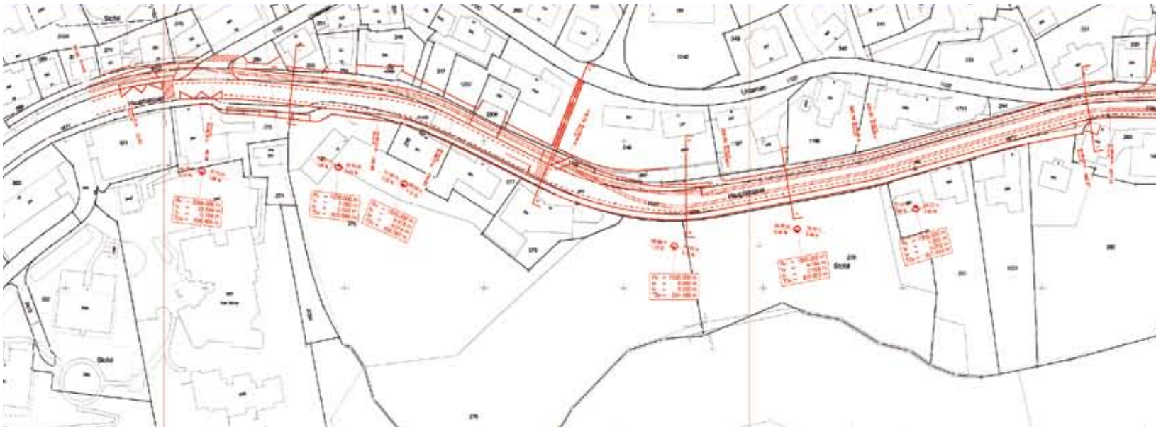
Situationsplan der Tram-Doppelspur: Vom Stofel bis zum Bahnhof sollen neu zwei Gleise in die Strasse verlegt werden.
